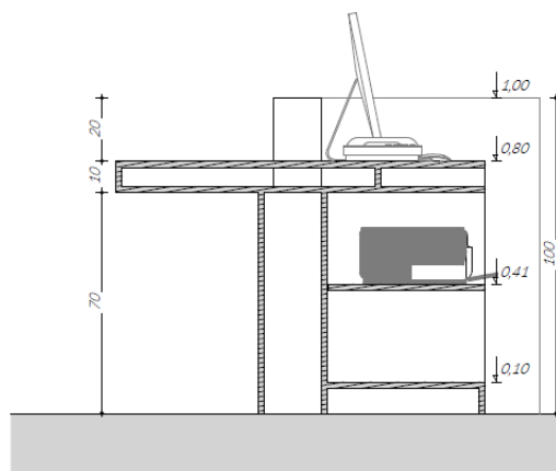
Coupe F - échelle 1/20°
